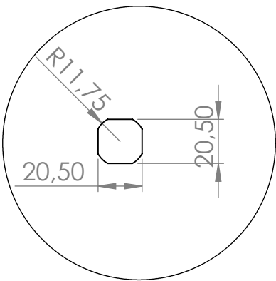
DÉTAIL A ECHELLE 2 : 5
