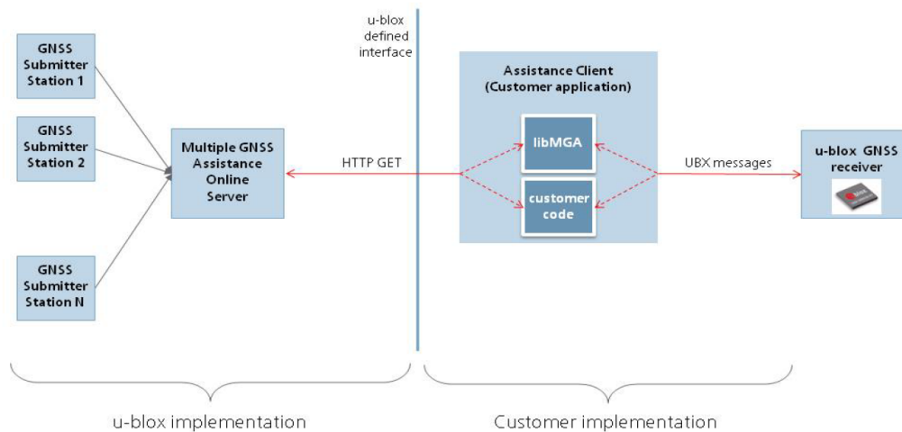
Figure 18: MGA architecture
